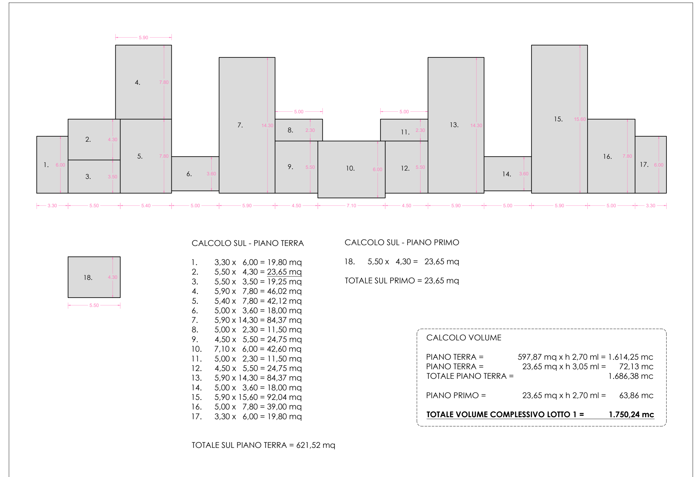
SCHEMA CALCOLO VOLUME Scala 1:200
