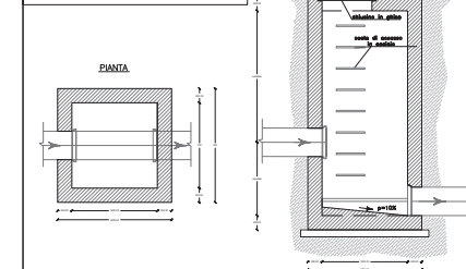
PARTICOLARE TIPO POZZETTO DI SALTO 120x120 ISPEZIONABILE
