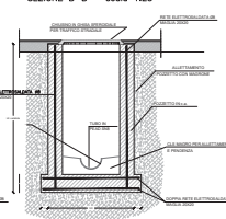
SEZIONE B-B - scala 1:25
