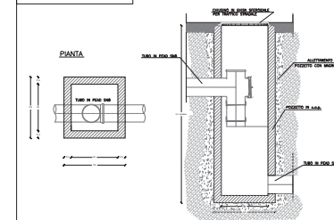
PARTICOLARE TIPO POZZETTO DI SALTO 80x80
