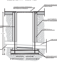
SEZIONE A-A - scala 1:25
