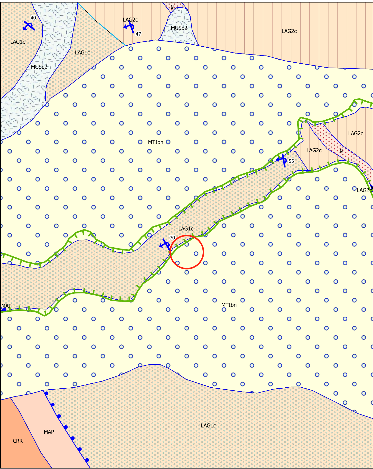
CARTA GEOLOGICA Scala 1 :5.000
