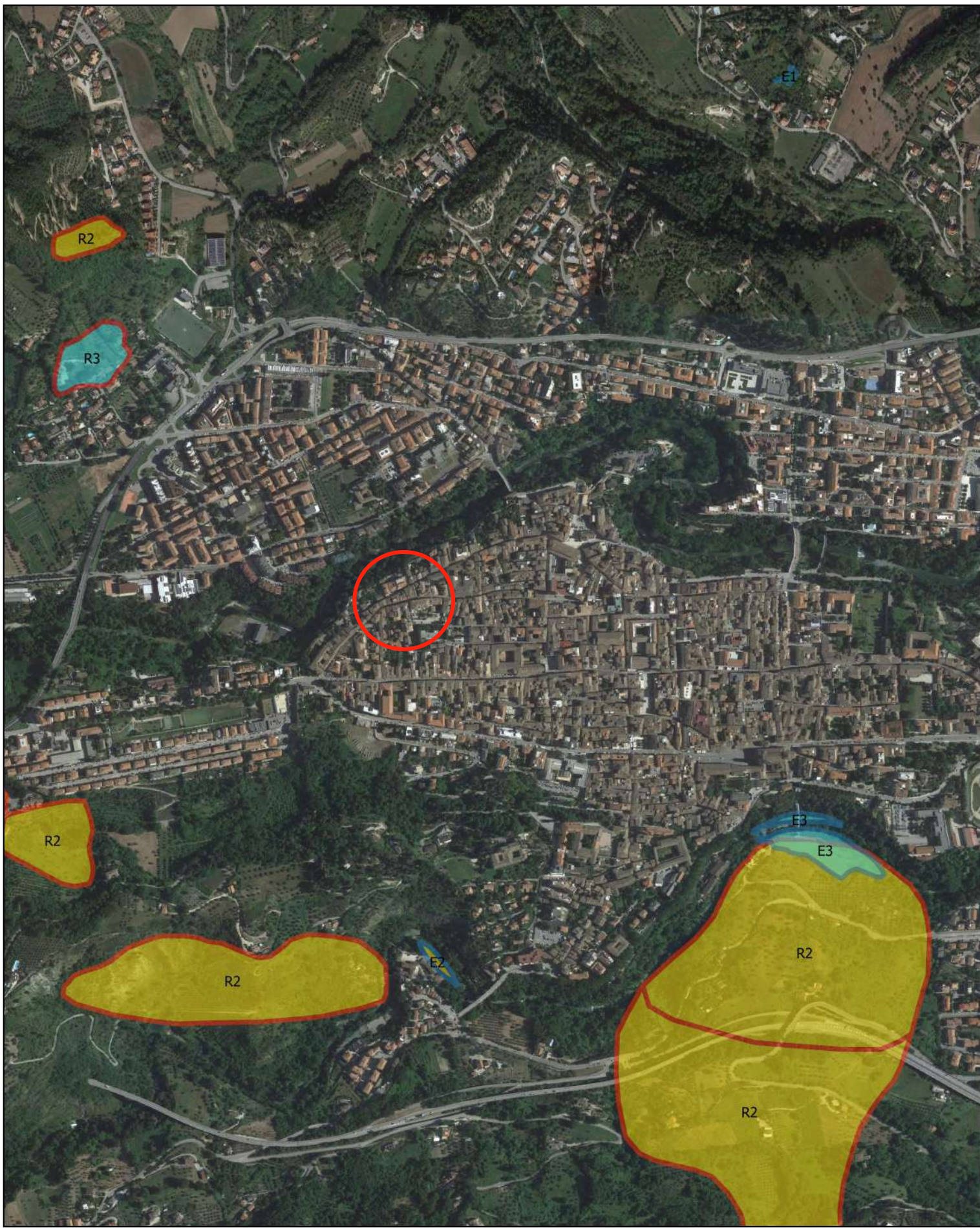
STRALCIO PAI TRONTO Scala 1 :10.000
