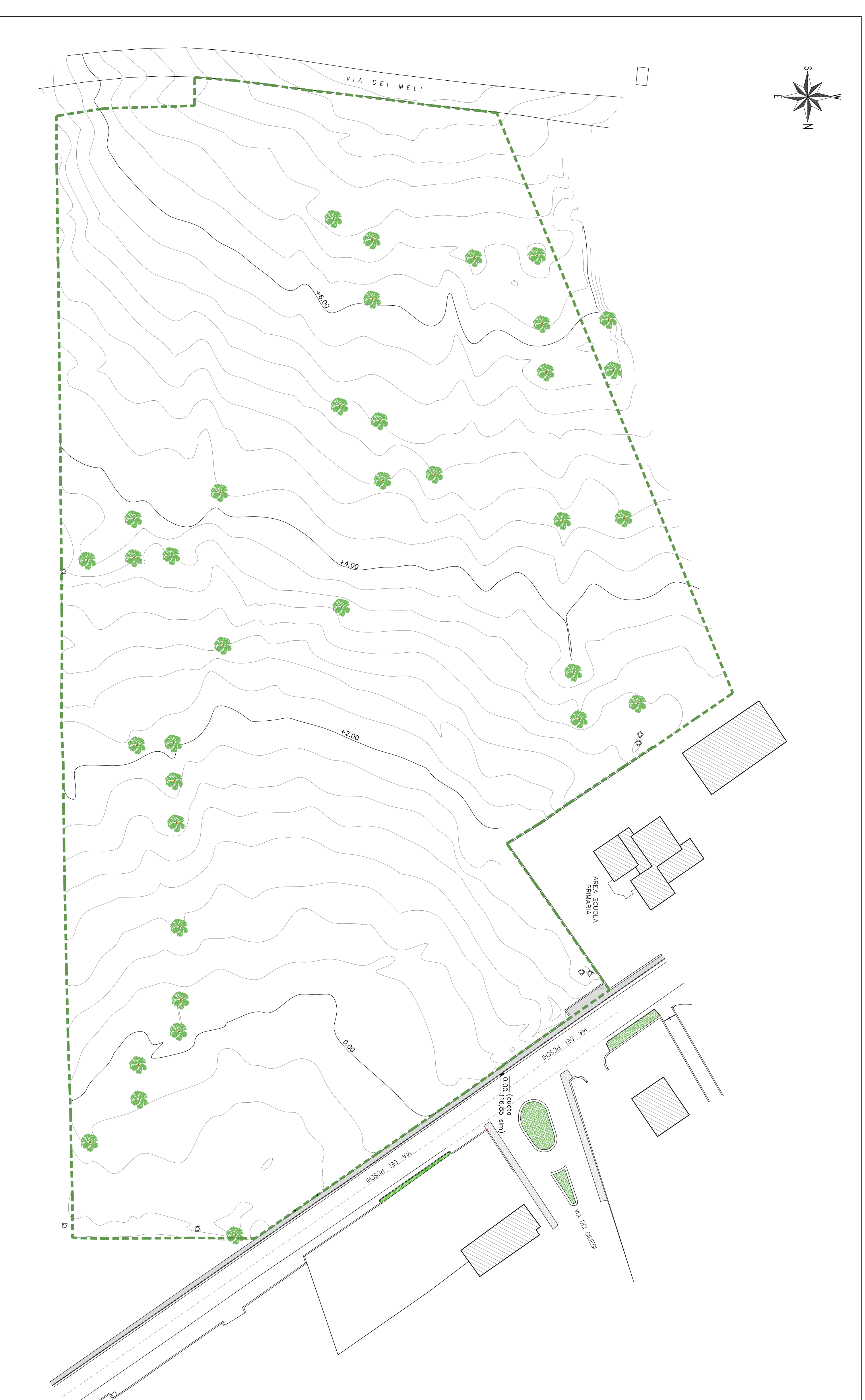
RILIEVO TOPOGRAFICO - scala 1:500
