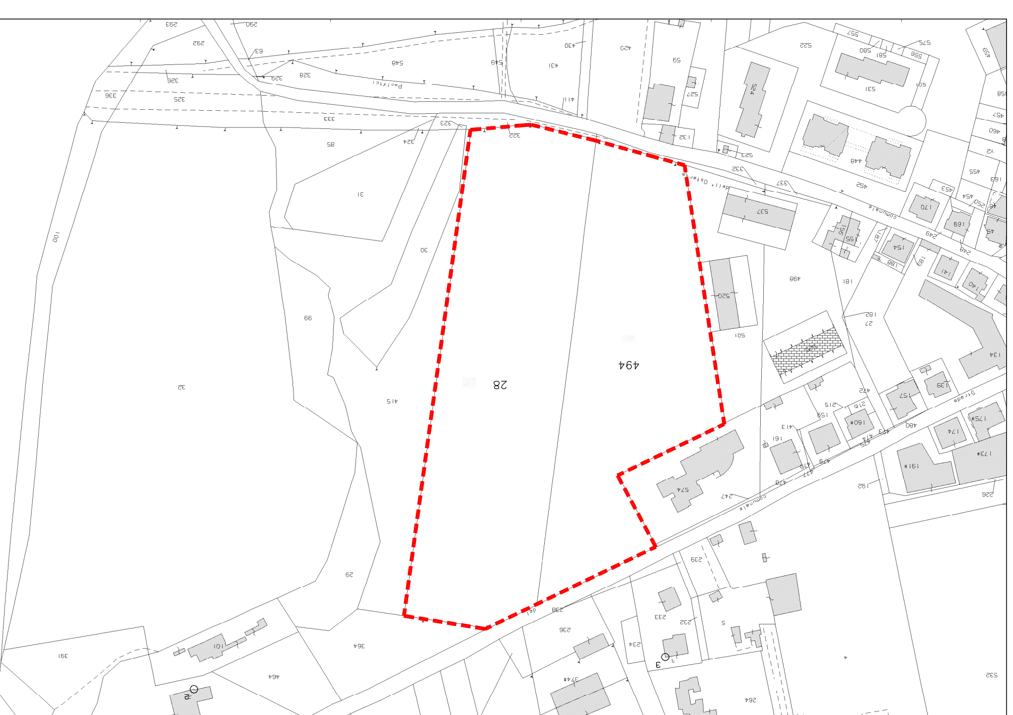
PLANIMETRIA CATASTALE - scala 1:2000 Foglio 111 - part. 28 e 494 LIMITE PROPRIETÀ BUILD S.R.L.
