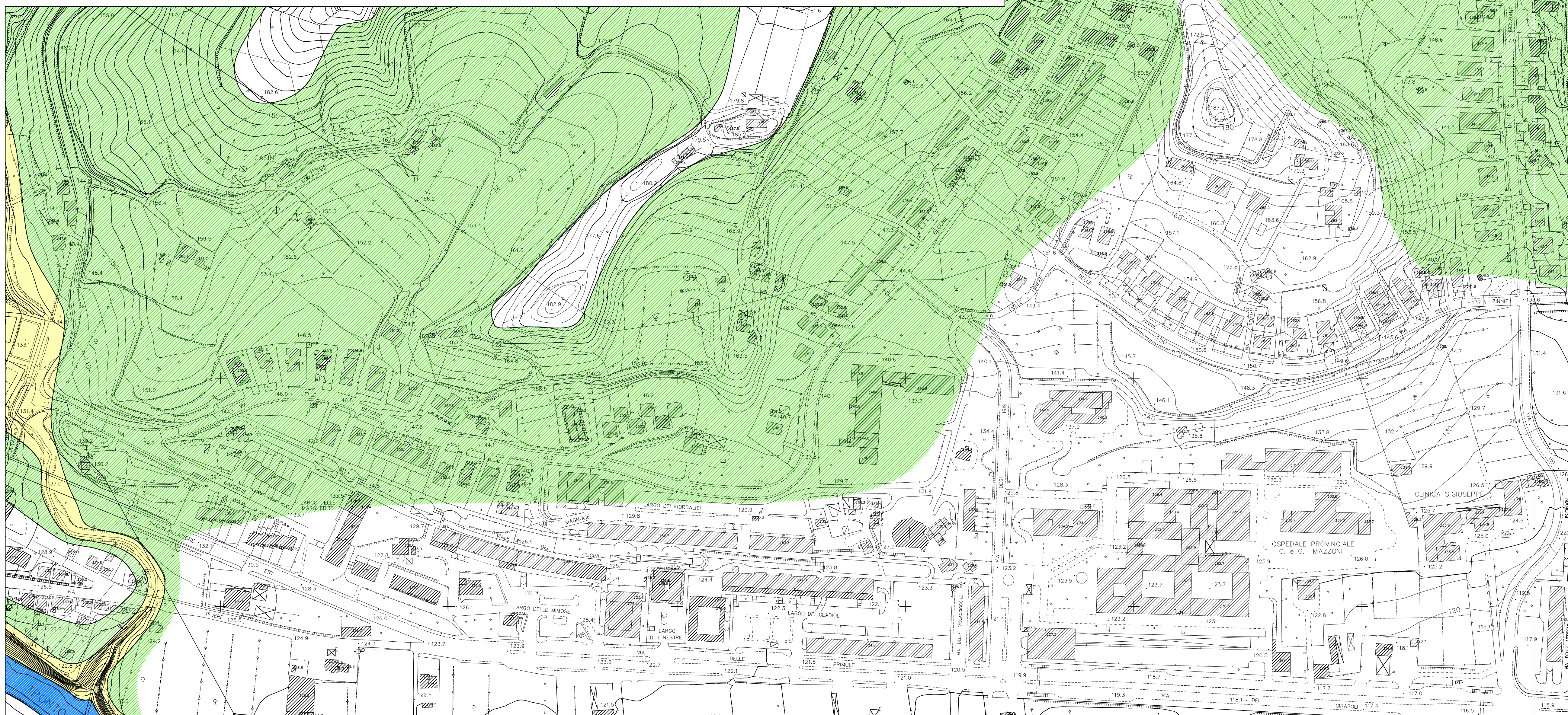
CARTA DELLE PERICOLOSITA' GEOLOGICHE Scala 1:2.000
